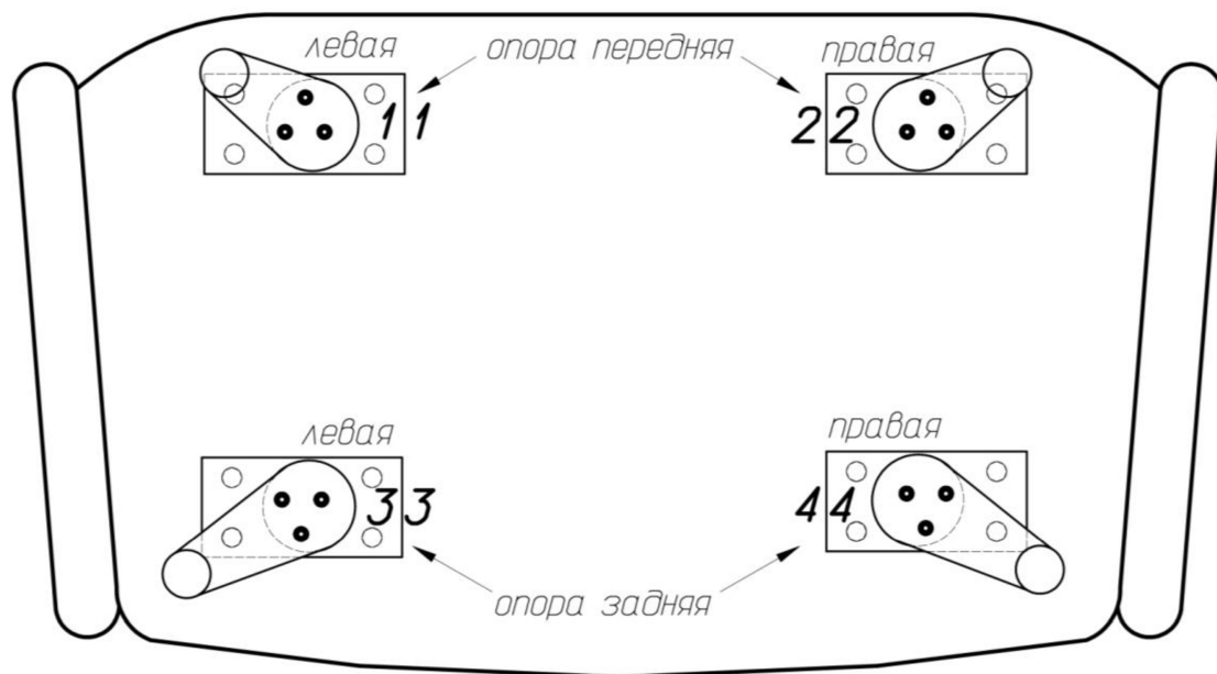
Схема установки опор
